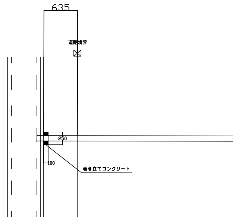
接続平面図
